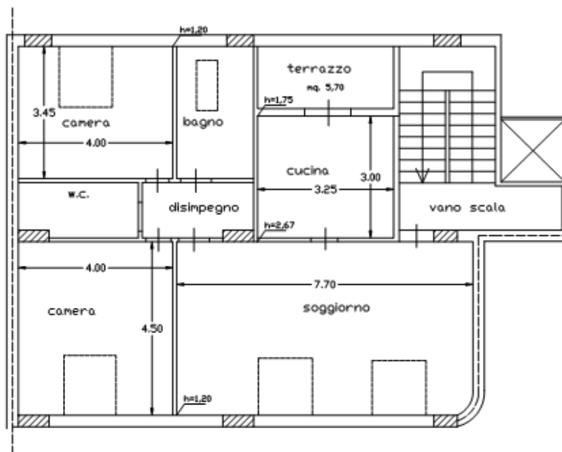
PIANTA PIANO QUARTO mansardato fg. 127 part. 321 sub 47
