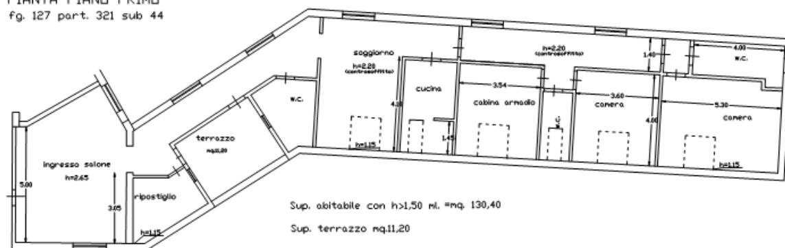
PIANTA PIANO PRIMO fg. 127 part. 321 sub 44
